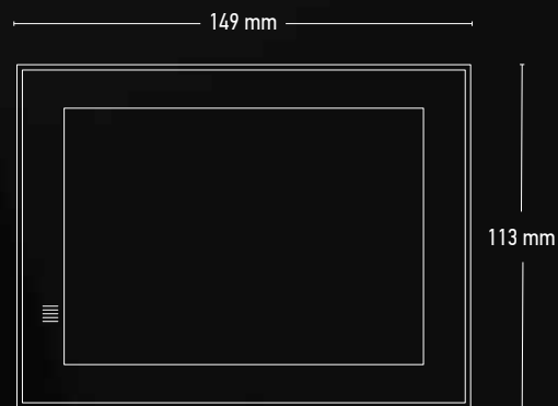
Πλαίσιο για χωνευτή τοποθέτηση
