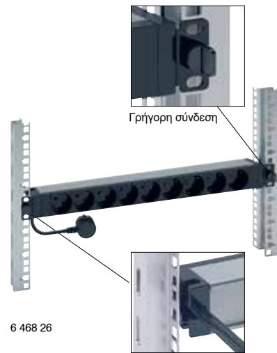
Ακραίο κάλυμμα με υποδοχή συγκράτησης καλωδίου
